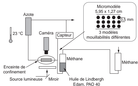
Figure 5 Montage expérimental pour la visualisation d’écoulements en micromodèles sous haute pression (Bora, Maini et Chakma, 1997).
